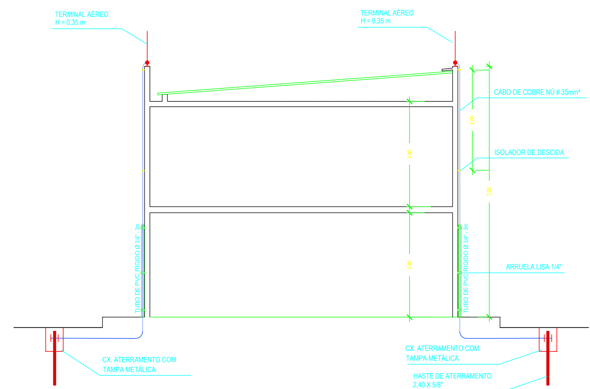
CORTE TRANSVERSAL ESQUEMÁTICO SEM ESCALA
