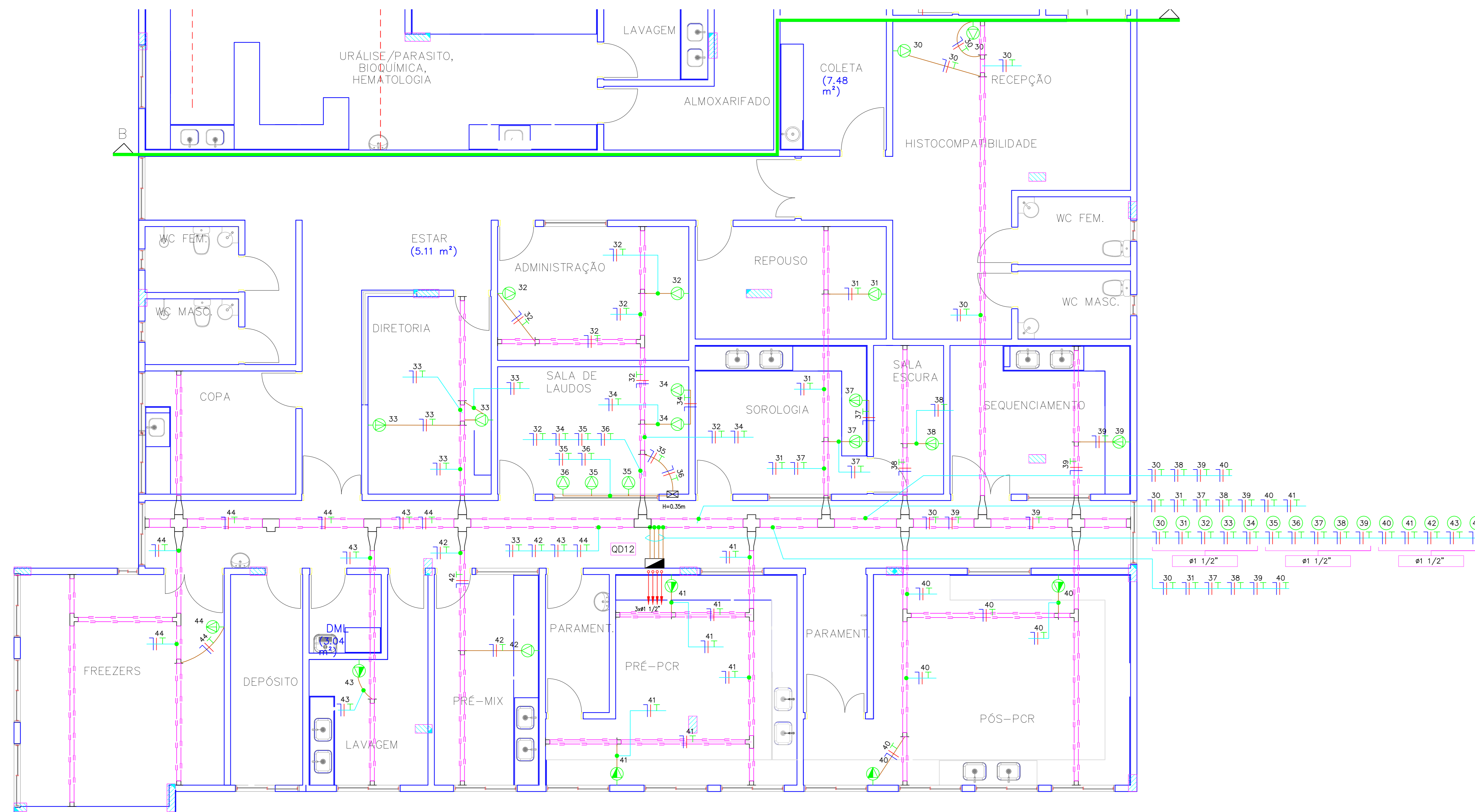
PLANTA BAIXA -1º Pavimento - Tomadas Computador ESCALA: 1 / 50
