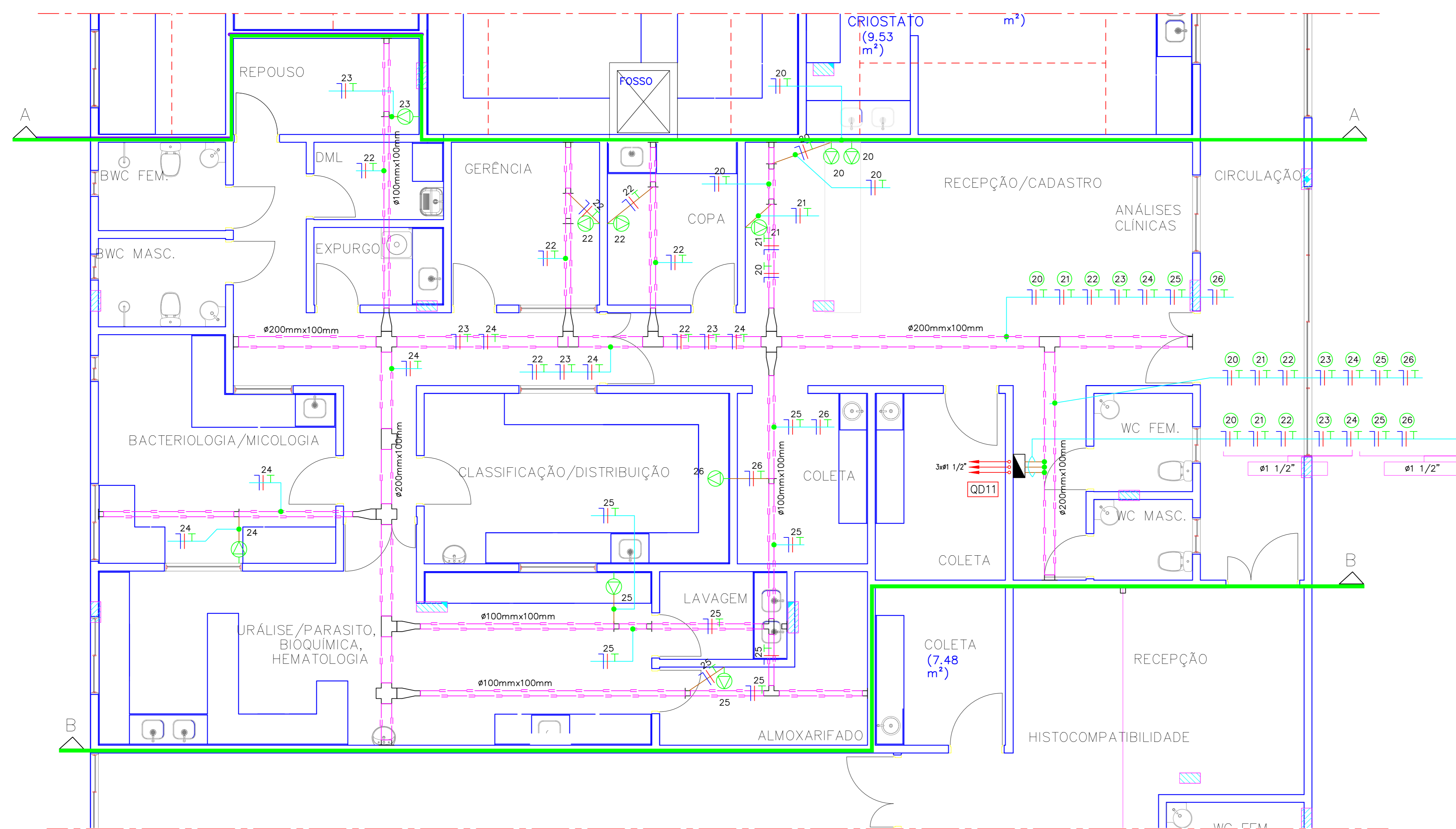
PLANTA BAIXA -1º Pavimento - Tomadas Computador ESCALA: 1 / 50
