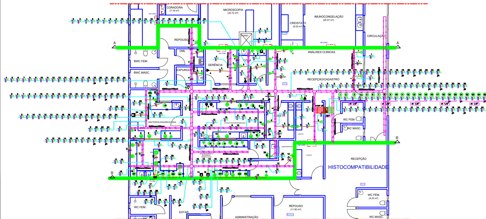
PLANTA BAIXA -1º Pavimento - Iluminação ESCALA 1:100
